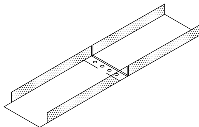
طريقه اتصال قطعات ۲متری سيني کابل
